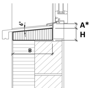
Querschnitt
