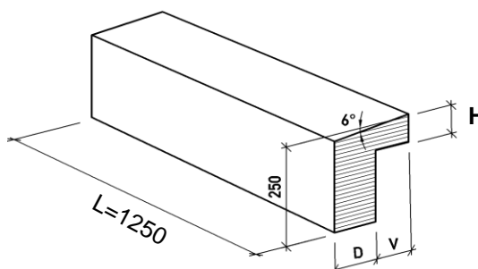
Isometrie
