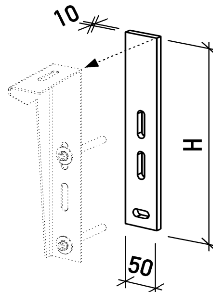
Thermostop Typ TSP * (selbstklebend) zu Typ MS Spezial
