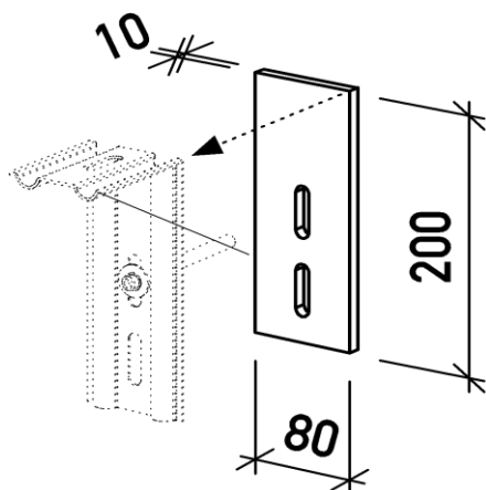
Thermostop Typ TSF * (selbstklebend) zu Typ MF, MR und MFA
