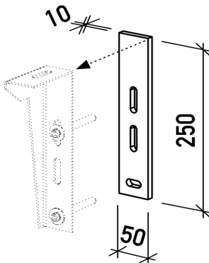
Thermostop Typ TSS * (selbstklebend) zu Typ MS
