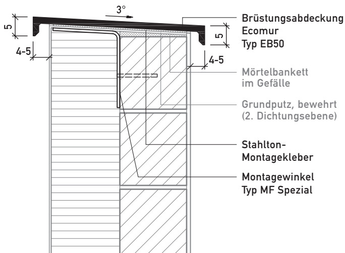
Typ EB50 Vertikalschnitt
