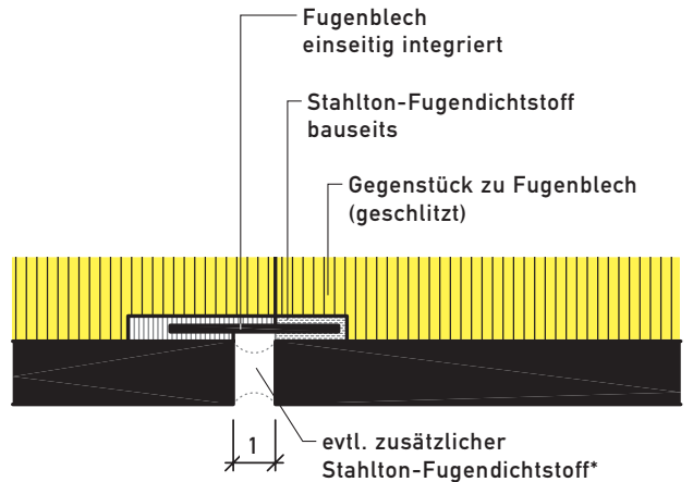
Horizontalschnitt Fugenausbildung 1:2 Typ EBJ
