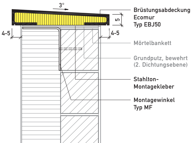
Typ EBJ50 Vertikalschnitt
