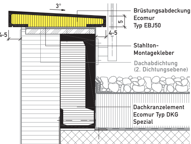
Ecomur Typ EBJ50 Vertikalschnitt
