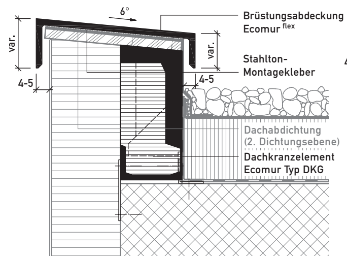
Ecomur flex Vertikalschnitt
