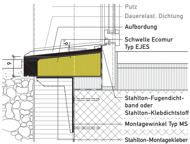
Typ EJES mit Aufbordung Vertikalschnitt
