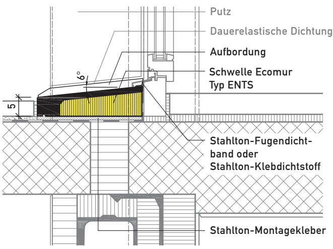
Typ ENTS mit Aufbordung Vertikalschnitt
