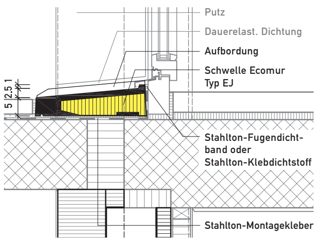
Typ EJ mit Aufbordung Vertikalschnitt
