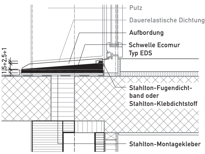
Typ EDS mit Aufbordung Vertikalschnitt
