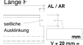
Draufsicht Fensterbank Länge F
