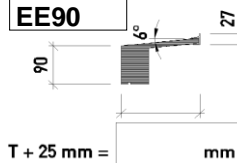
Fensterbank Typ EE90
