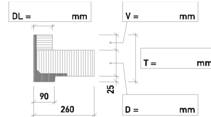
Fensterbank Typ EE90
