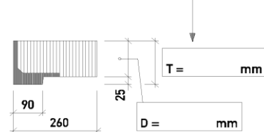
Fensterbank Typ EE90
