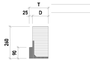
Sturzverkleidung Typ VD90
