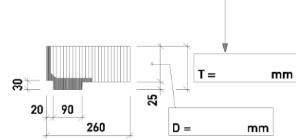
Fensterbank Typ EE90
