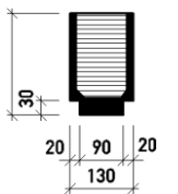
Draufsicht Fensterbank Länge F
