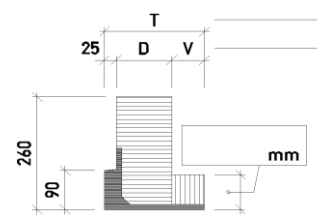
Sturzverkleidung Typ V90
