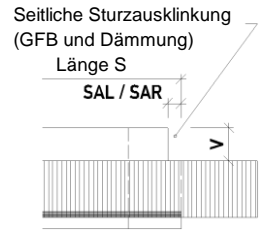
Grundriss G-G
