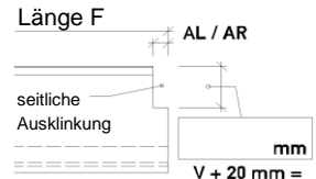
Draufsicht Fensterbank
