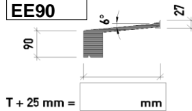
Fensterbank Typ EE90
