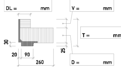
Fensterbank Typ EE90
