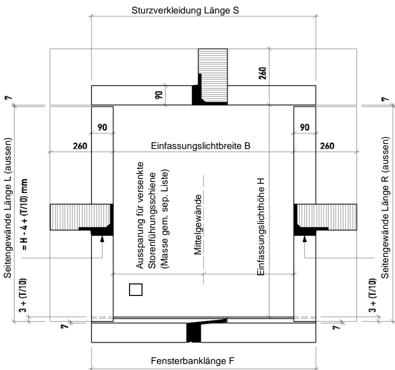
Ansicht von aussen
