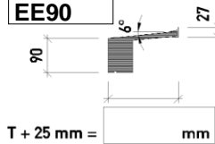
Fensterbank Typ EE90
