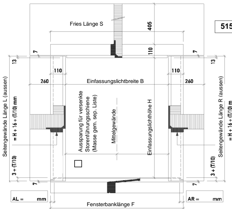
Ansicht von aussen
