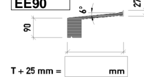
Fensterbank Typ EE90
