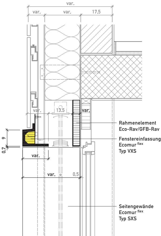
Vertikalschnitt durch Fenster
