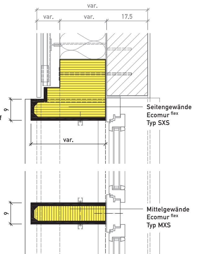
Horizontalschnitt durch Gewände
