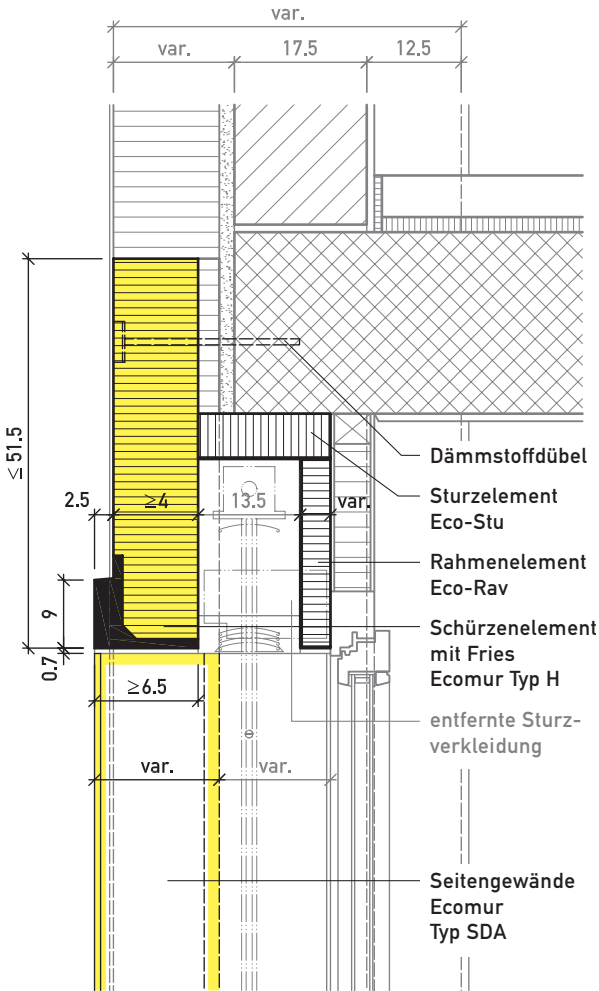
Vertikalschnitt durch Fenster
