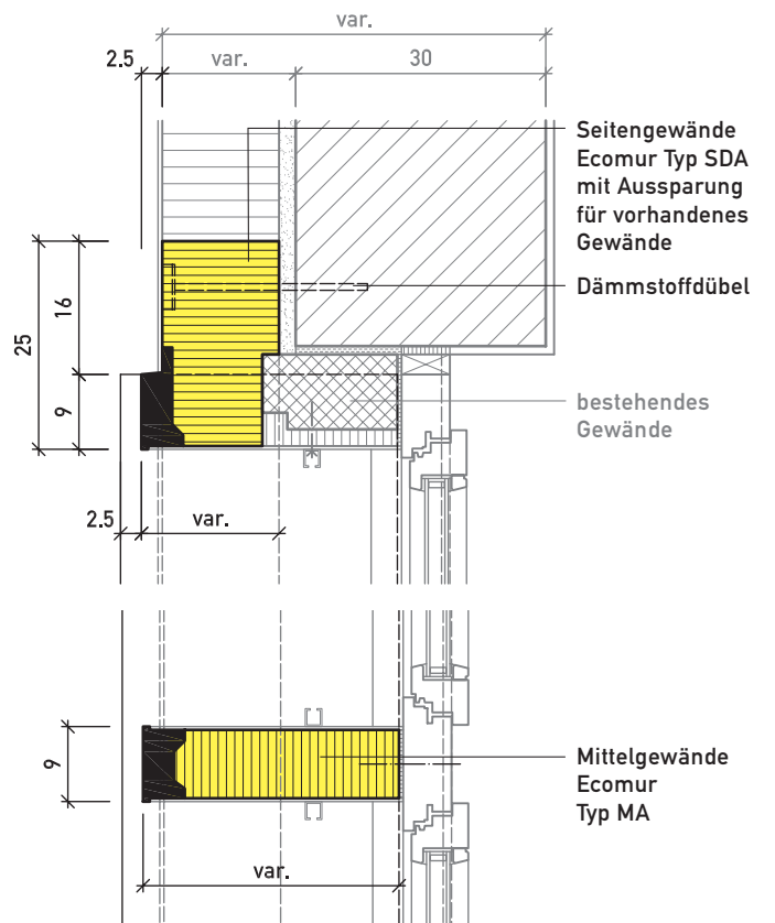
Horizontalschnitt durch Gewände
