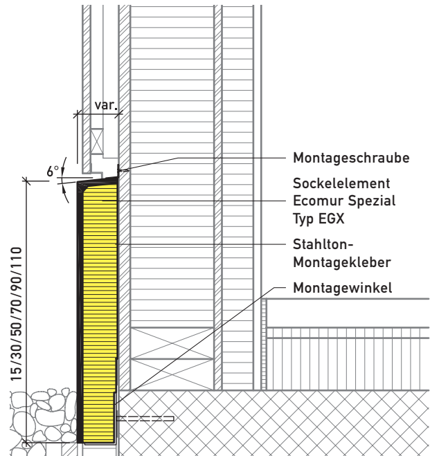
Hinterlüftete Fassade Vertikalschnitt Ecomur Spezial
