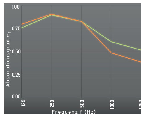
Valeurs de mesure EMPA, panneaux Mock-up, isolation en laine de roche 200 mm, taux de surface perforée 24 %
