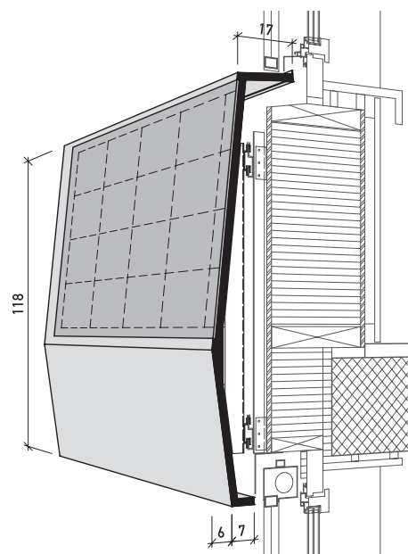
Coupe à travers la fenêtre
