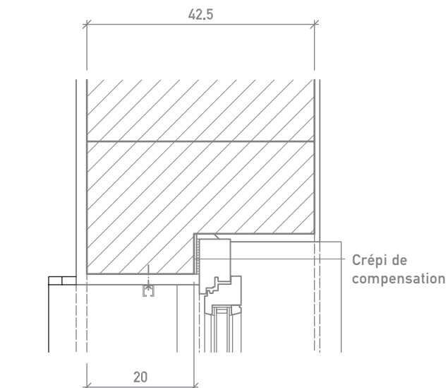
Coupe horizontale de l'embrasure
